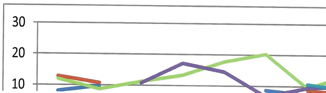
Fig. nr. 3: Evoluția concentrației medii anuale (în \mu\text{g}/\text{m}^3 ) pentru \text{SO}_2 în perioada 2011 – 2021
