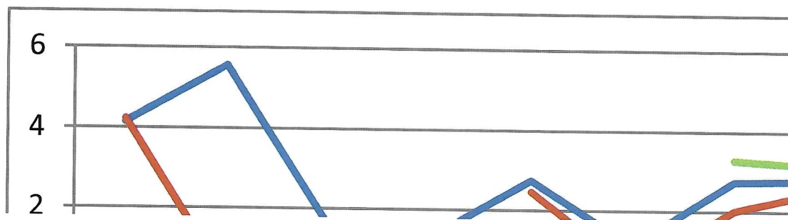
Fig. nr. 5: Evoluția concentrației medii anuale (în \mu\text{g}/\text{m}^3 ) pentru benzen în perioada 2011 – 2021
