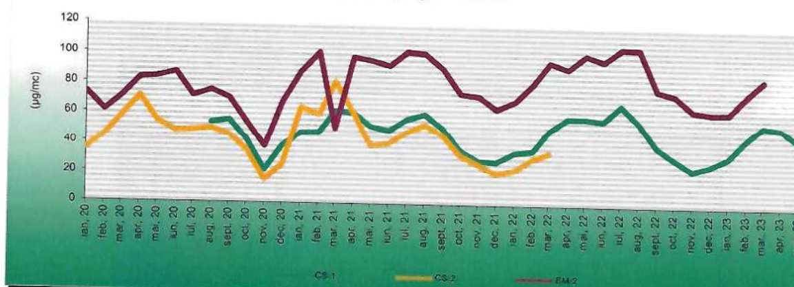
Concentrații O 3 medii lunare
