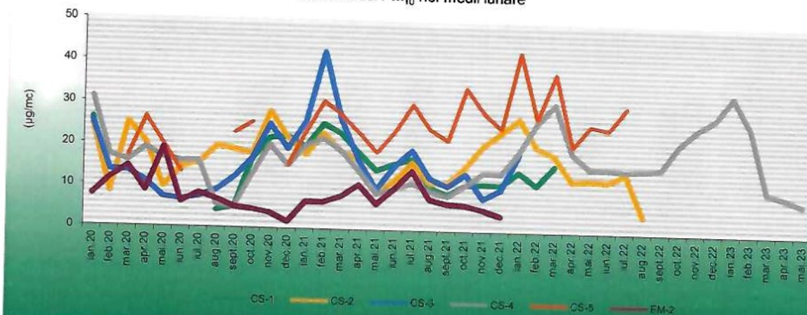
Concentrații PM 10 nef medii lunare
